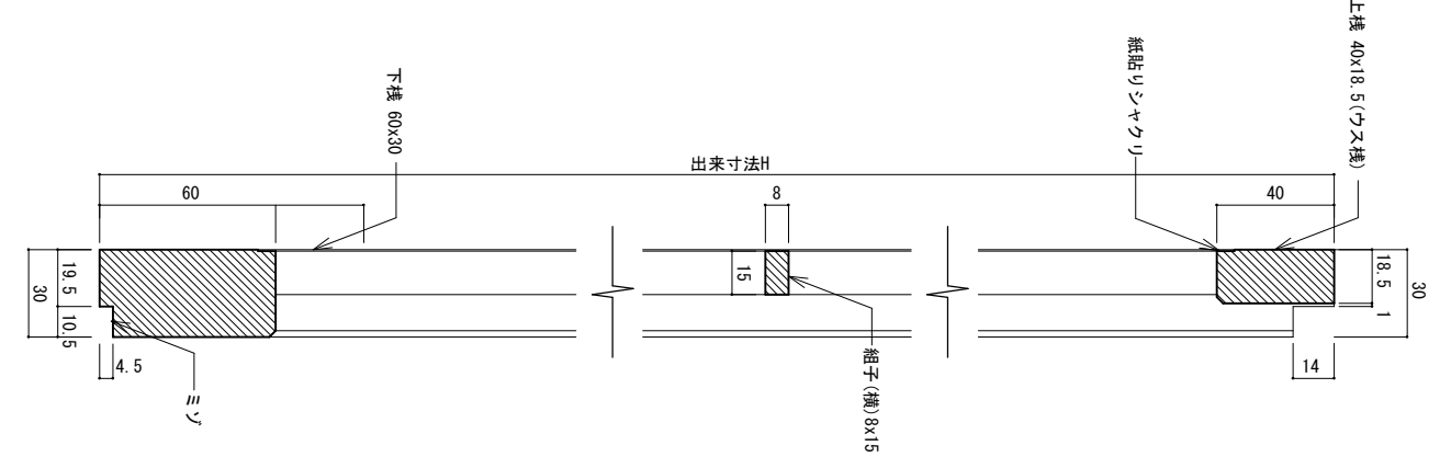
縦断面詳細図 S:1/2
