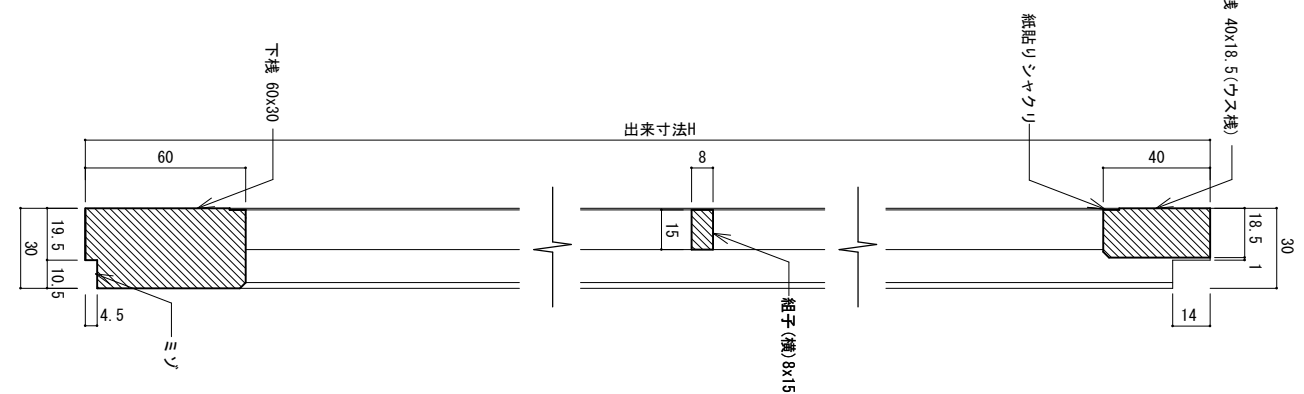
縦断面詳細図 S:1/2
